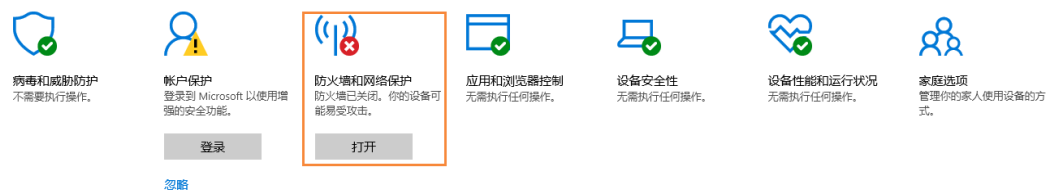
图4-3 防火墙
