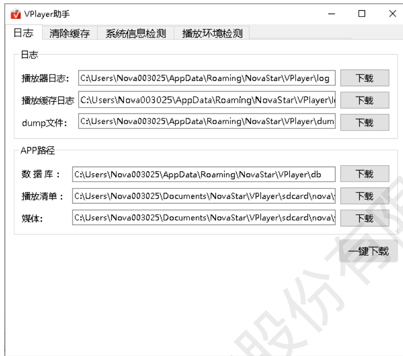
图5-2 VPlayer 助手
