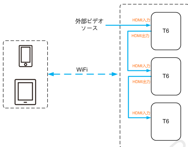
図3-10 デバイス接続例
