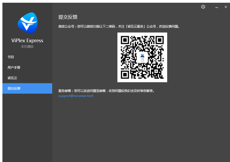
图6-2 启动页菜单
