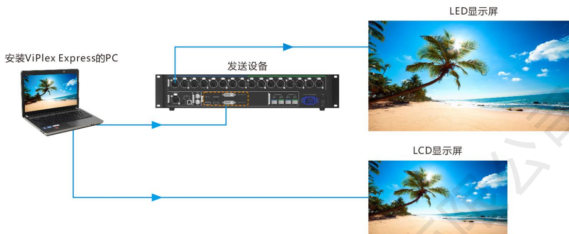
图2-8 连接显示屏
