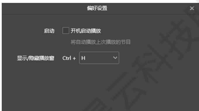
图6-1 偏好设置
