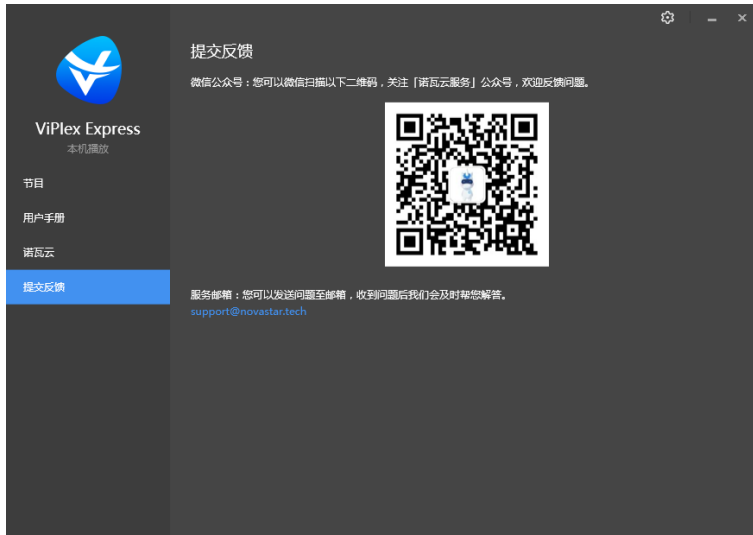
图6-4 启动页菜单
