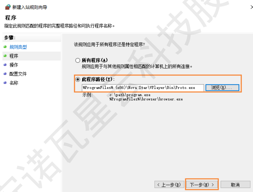
图6-4 选择程序
