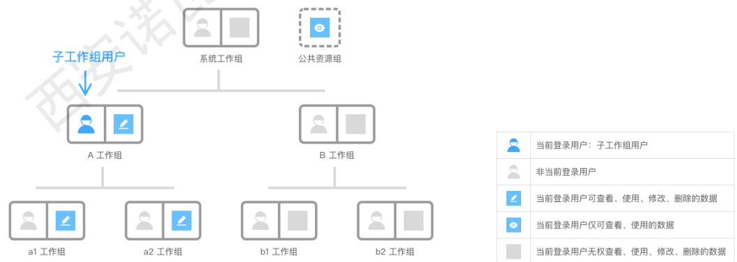
图3-4 数据操作权限—子工作组用户
