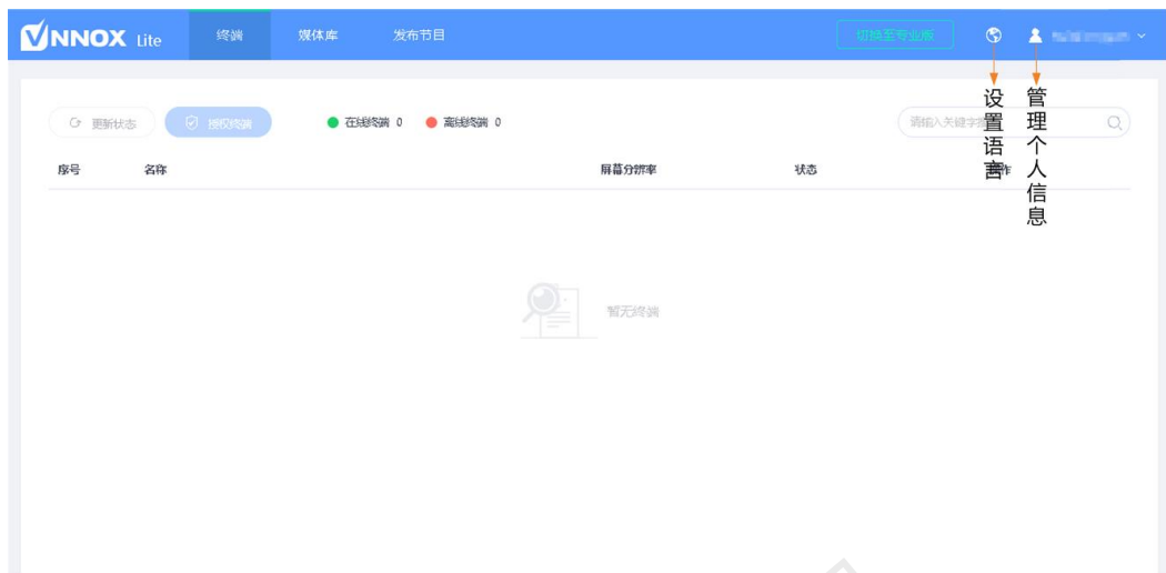
图3-1 简易版界面
