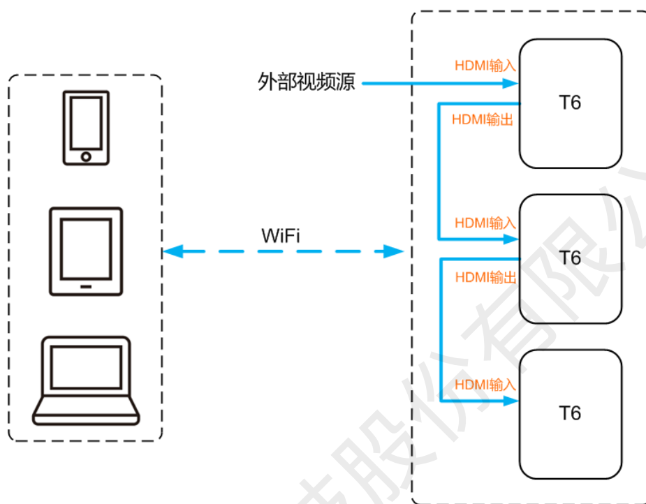
图4-1 终端连线示例
