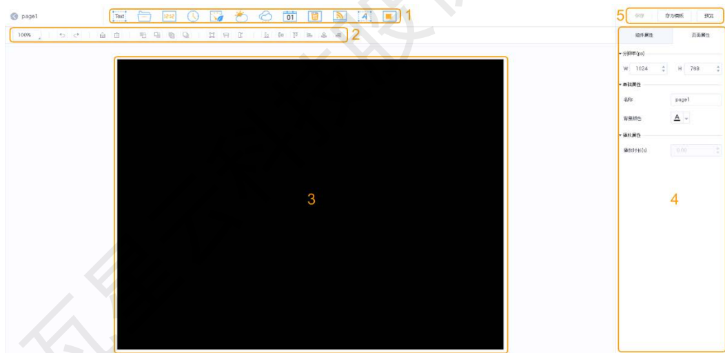
图3-1 编辑界面
