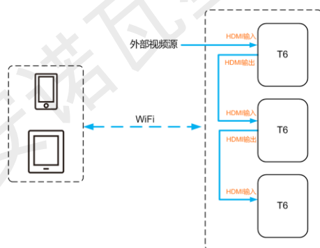
图3-10 设备连线示例
