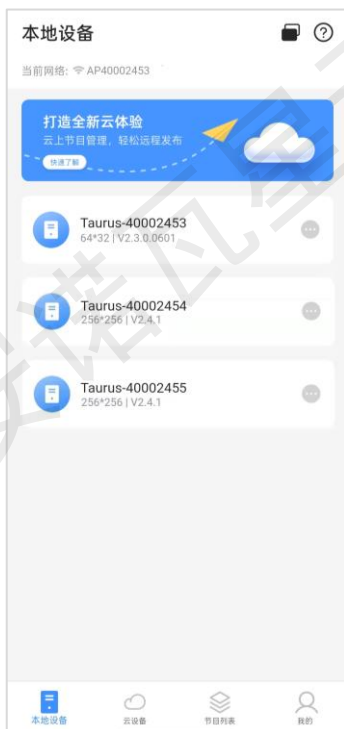
图3-12 本地设备
