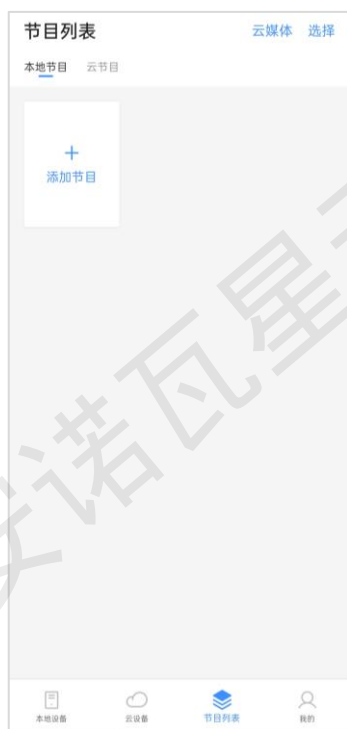
图5-1 本地节目
