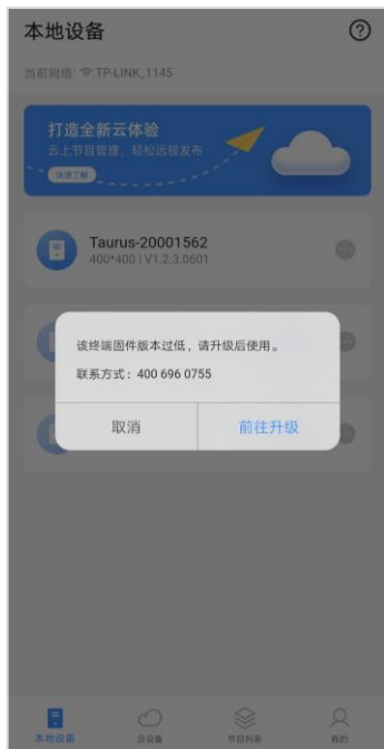
图7-1 界面提示
