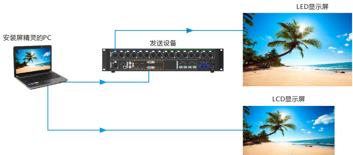
图2-8 连接显示屏
