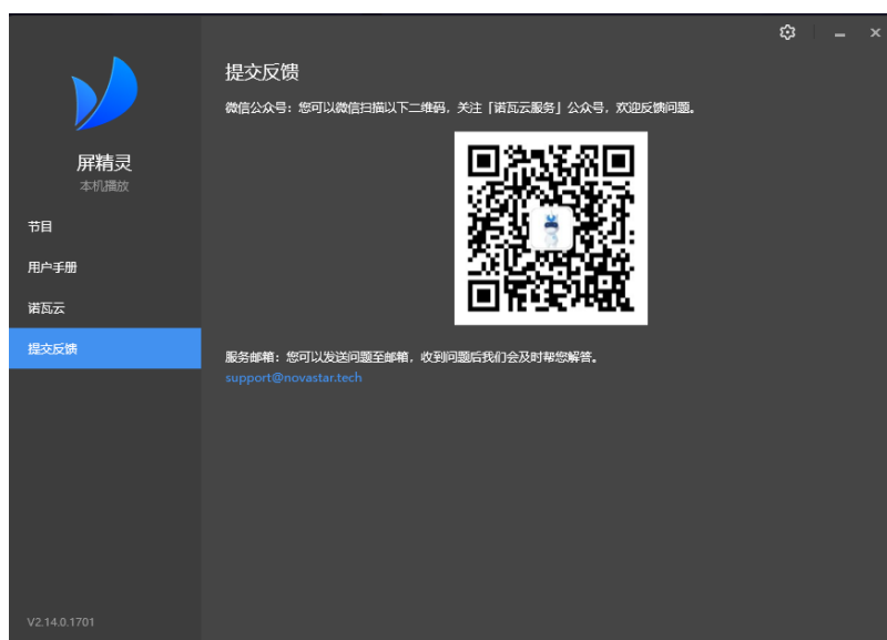
图6-2 启动页菜单
