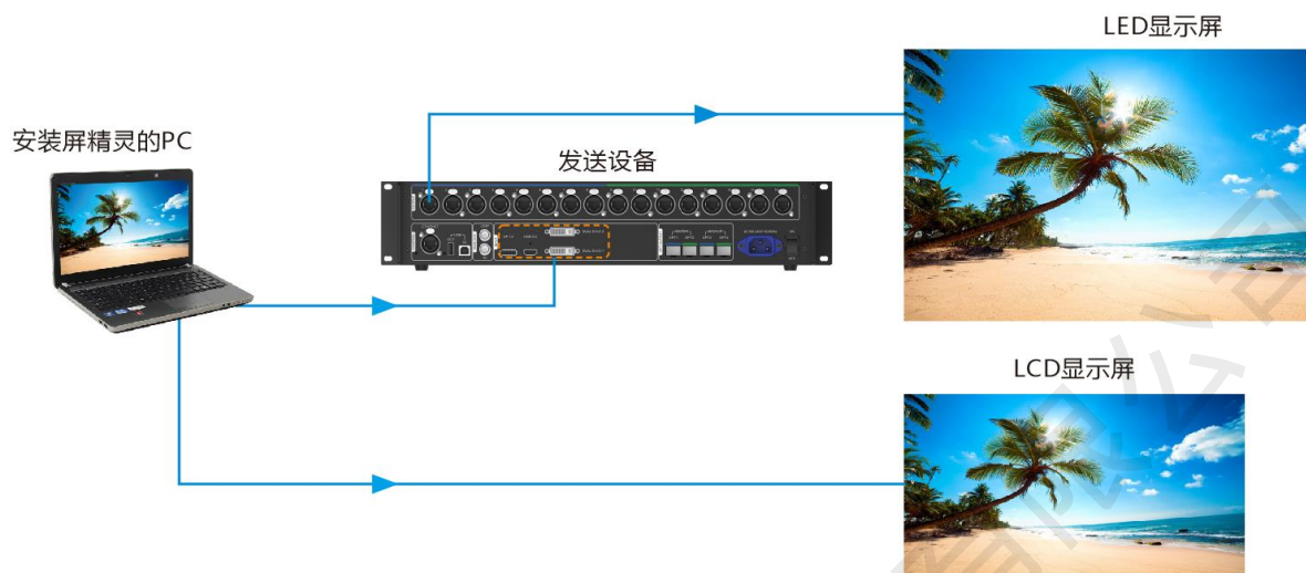
图2-8 连接显示屏
