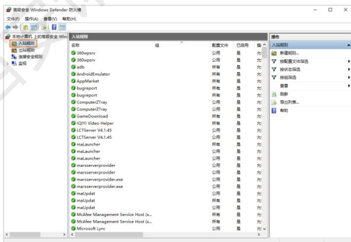
图7-2 入站规则
