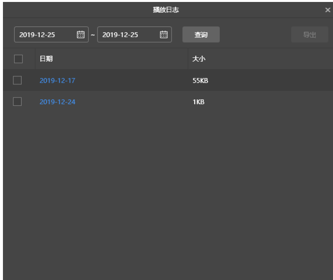
图5-2 查询结果
