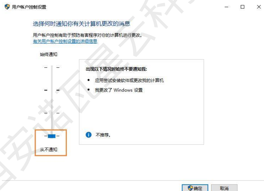
图2-5 UAC
