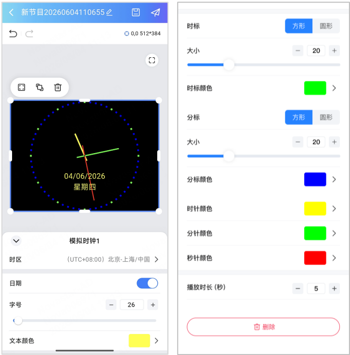
图3-13 设置媒体属性
